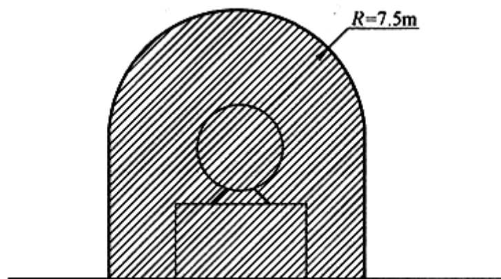
图B.0.14 露天（棚）设置的天然气压缩机组、阀门、法兰或类似附件的爆炸危险区域划分 距压缩机、阀门、法兰或类似附件的壳体 7.5m 以内并延至地面的空间划为 2 区。
