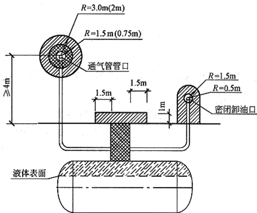
图8.0.5 埋地卧式汽油储罐爆炸危险区域划分
