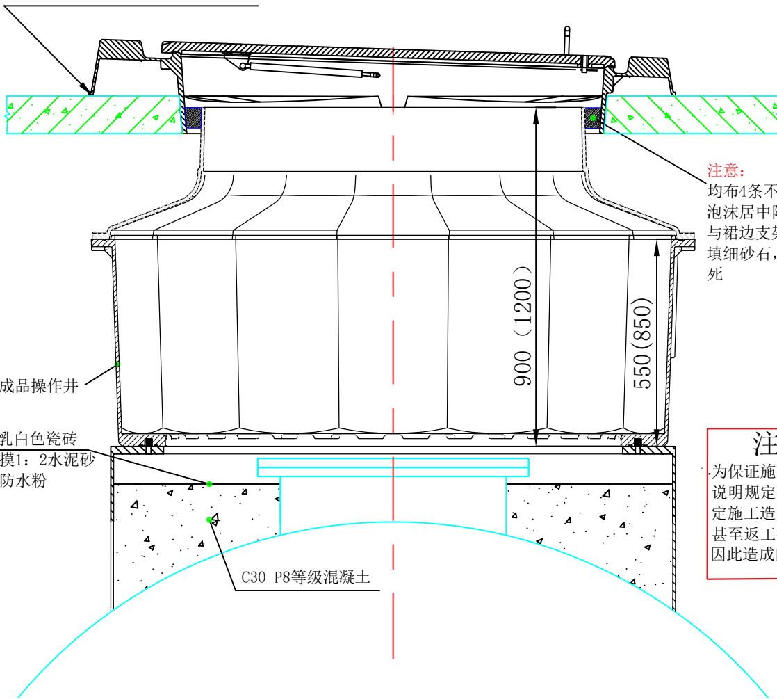
非承重油罐操作井做法图
